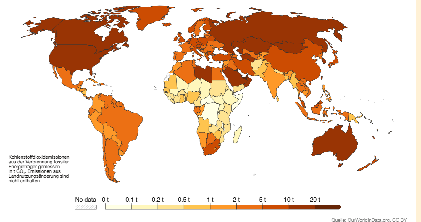
CO 2 -AUSSTOSS PRO KOPF WELTWEIT NACH LÄNDERN, 2021
