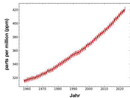
ATMOSPHÄRISCHES CO 2 AM MAUNA-LOA-OBSERVATORIUM
