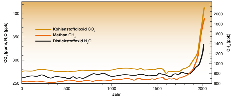
ATMOSPHÄRISCHE KONZENTRATION WICHTIGER TREIBHAUSGASE 0-2022
