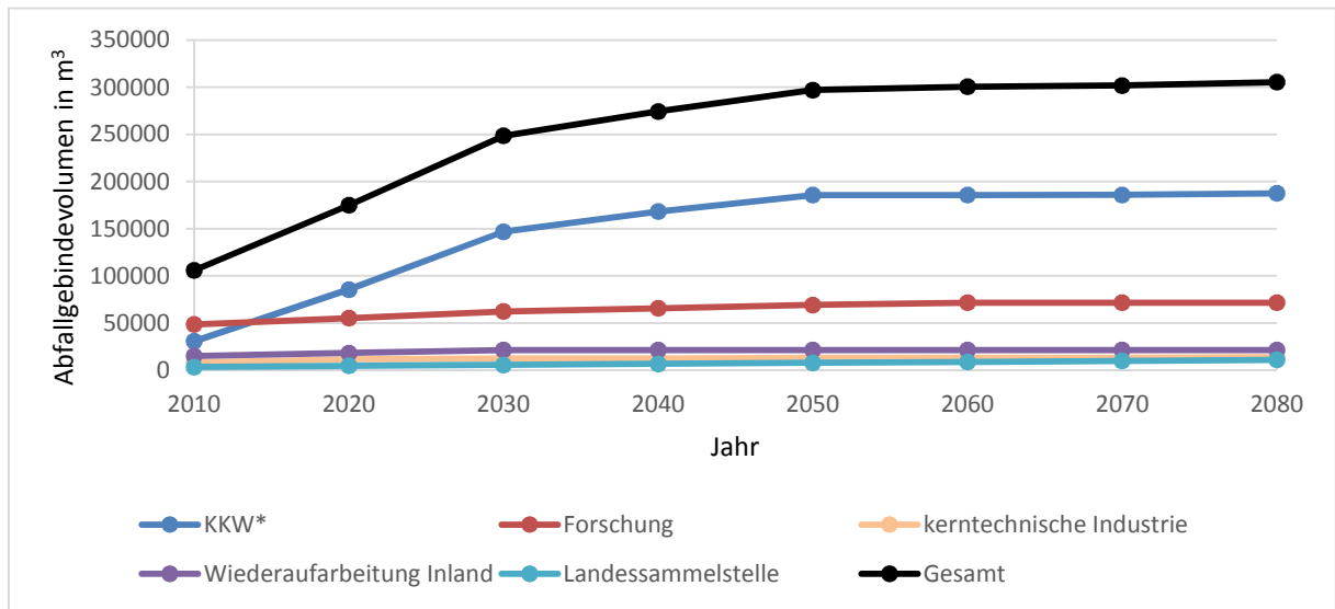
Abbildung 2.2: Zeitlicher Verlauf des kumulierten Anfalls radioaktiver Abfälle mit vernachlässigbarer Wärmeentwicklung als Abfallgebundevolumen bis zum Jahr 2080
