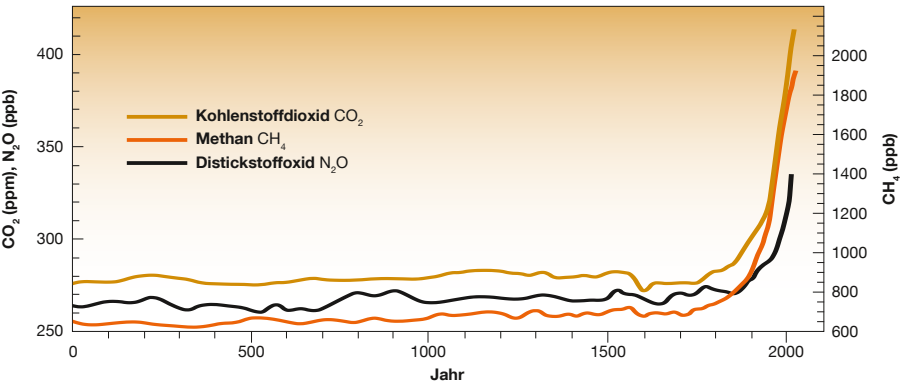
ATMOSPHERISCHE KONZENTRATION WICHTIGER TREIBHAUSGASE 0-2022
