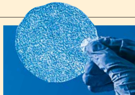
Jahresscheibe aus einem Antarktis-Eisbohrkern mit eingeschlossenen Luftbläschen
