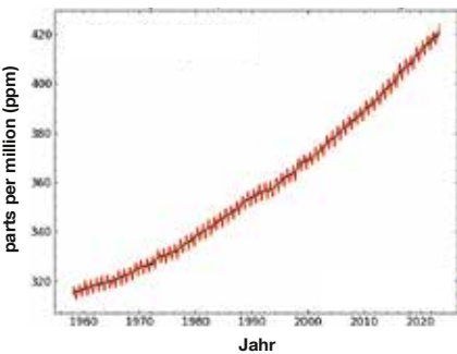
ATMOSPHERISCHES CO 2 AM MAUNA-LOA-OBSERVATORIUM
